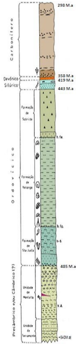
Fig. 7.3 - Coluna estratigráfica da região de Valongo adaptada de (COUTO, 1993)
