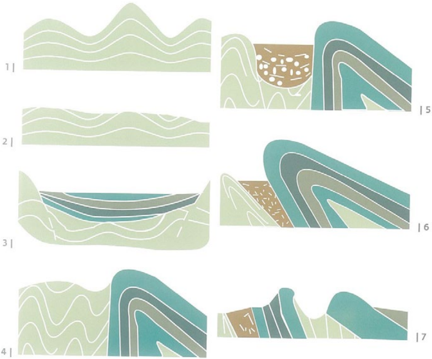
Fig. 7.2 - Evolução geotectónica do Anticlinal de Valongo (in Couto e Lourenço, 2011 (modificado de Couto, 1993)). 1-Atuação da tectónica que deformou as rochas do Precâmbrio e/ou Câmbrio. 2-Subsequente erosão destas rochas originando uma superfície de aplanamento. 3-Abertura de rifte originando um mar onde depositaram sedimentos desde o Ordovícico Inferior ao Devónico Inferior. 4-A tectónica atua de novo (1ª fase da orogenia Varisca) formando o Anticlinal de Valongo. 5-Bacias continentais instalaram-se numa zona intramontanhosa a oeste do flanco inverso. 6-Fases mais tardias da orogenia Varisca voltam a deformar as rochas provocando o tombamento do Anticlinal para oeste. 7-Os agentes erosivos transformam uma montanha num grande vale.
