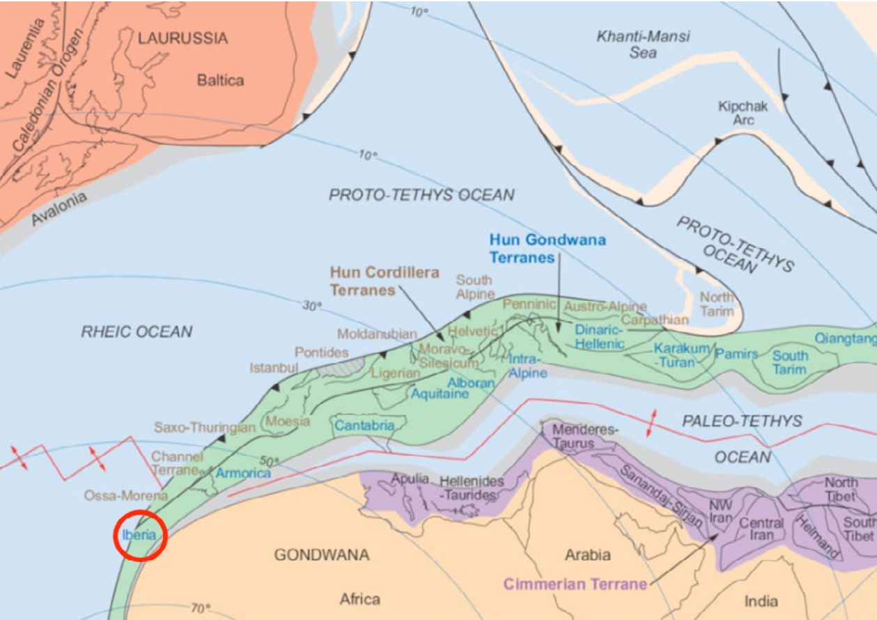
Fig. 7.1 - Reconstrução da tectónica de Placas com a localização a vermelho da localização da Iberia por altura do Silúrico (Stampfli et al. 2001)
